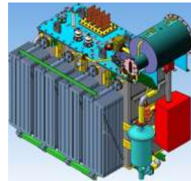
3D – модель трансформатора ЭОМНШ-2500/10
